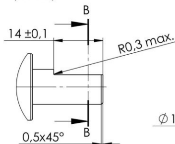
Detail A (2 : 1.5)
