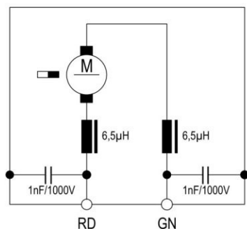
Schaltbild / circuit diagram
